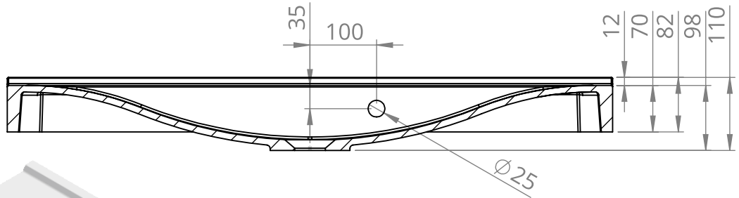
PRZEKRÓJ M-M SKALA 1 : 8
